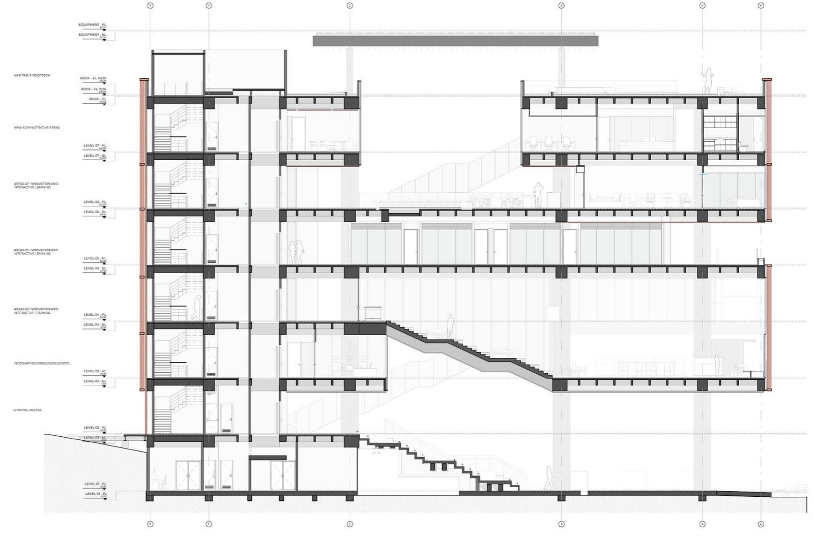
Sección B-B
